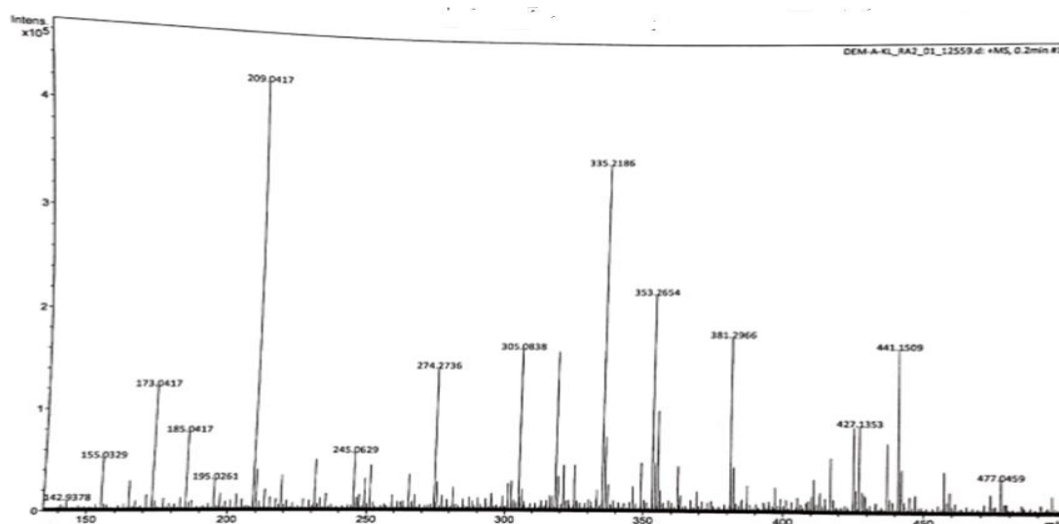
Fig. 7. ESI-MS spectrum of Kraft lignin
