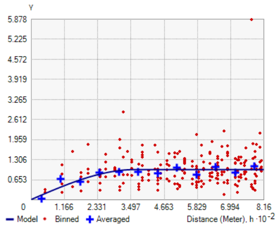
Available Cu
